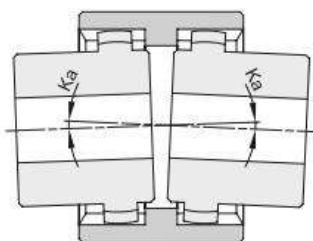
Угловое смещение
