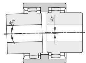
Угловое/Радиальное смещение
