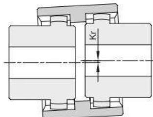
Радиальное смещение
