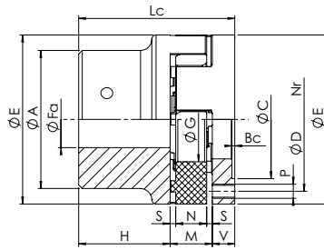
flange - shaft
