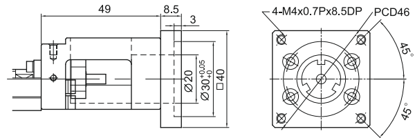
Модуль КК40 переходный фланец F1
