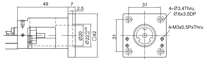
Модуль КК40 переходный фланец F3
