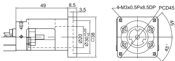
Модуль КК40 переходный фланец F2
