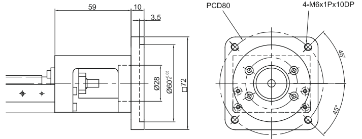
Модуль KK60 переходный фланец F9
