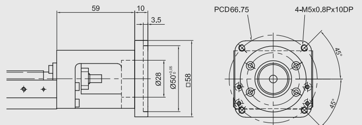
Модуль KK60 переходный фланец F11
