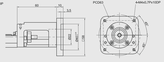
Модуль KK50 переходный фланец F7
