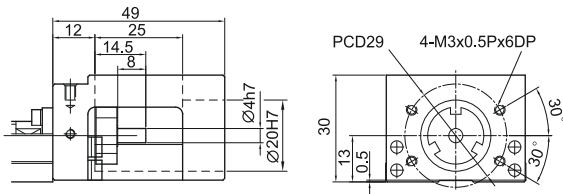
Модуль КК40 переходный фланец F0
