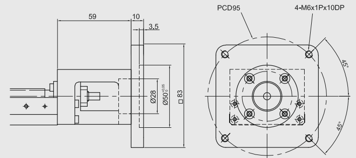
Модуль KK60 переходный фланец F9
