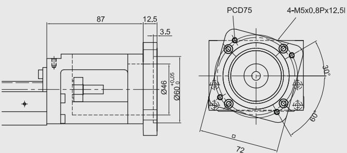
Модуль КК86 переходный фланец F10
