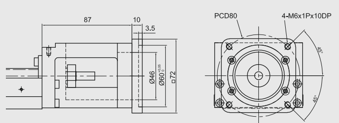
Модуль КК86 переходный фланец F9
