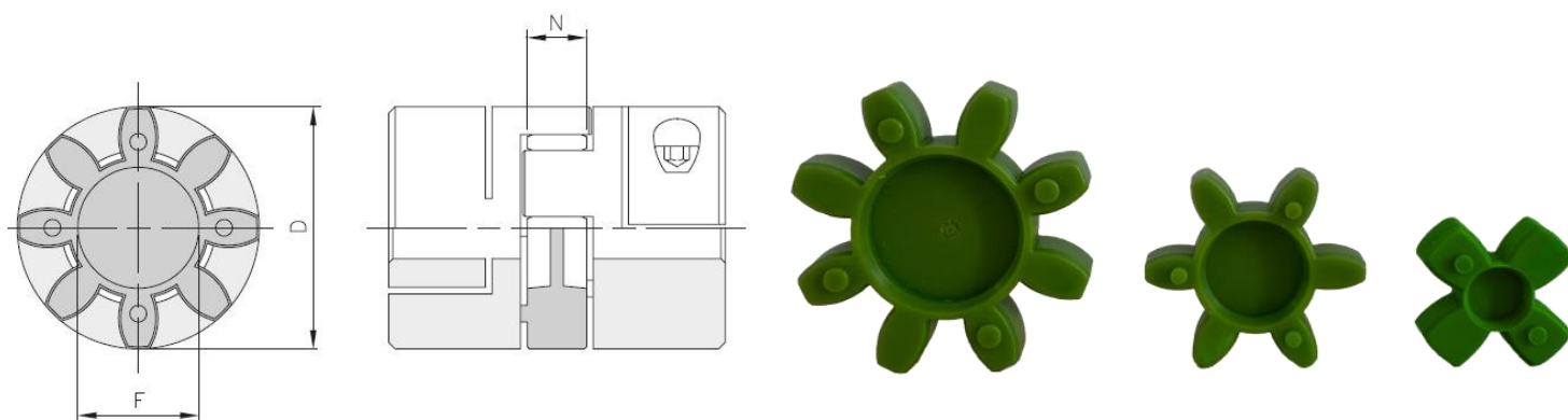
Эластичный зубчатый элемент из полиуретана (зеленый цвет) - "64 Shore D"
